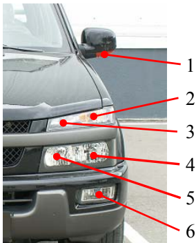
Рис. 37. Приборы передней световой сигнализации
