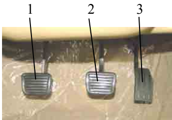
Рис. 44. Расположение педалей
