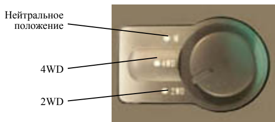
Рис. 56. Положение переключателя режимов раздаточной коробки без понижающей передачи
