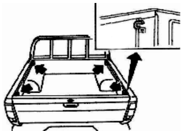
Рис. 58. Крепежные крюки грузовой платформы
