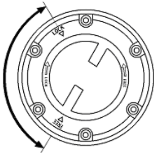
Рис. 57. Муфта включения привода переднего колеса
