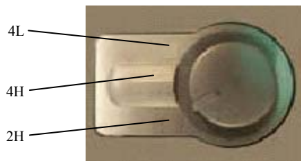
Рис. 55. Положение переключателя режимов раздаточной коробки с понижающей передачей
