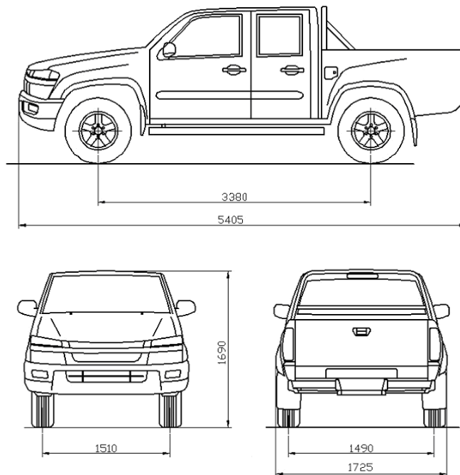
Рис. 1. Габаритные размеры автомобиля ДЕРВЕЙС – 2333
