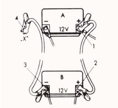
Рис. 66. Присоединение батареи
